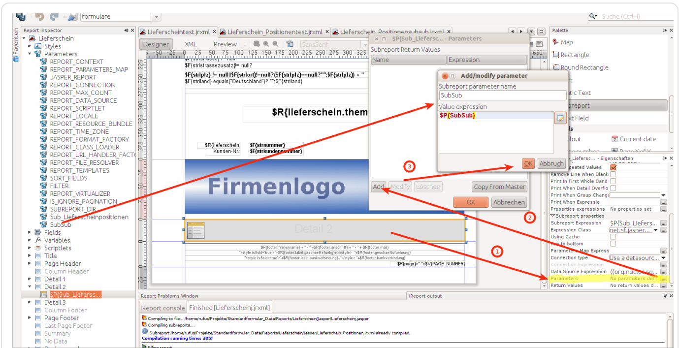
Parameter passing main sub subsub.
